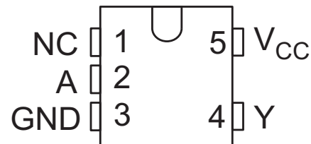
DCK 或 DBV 封装 (顶视图)
